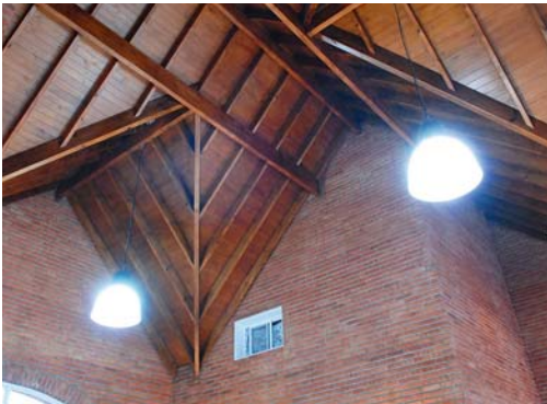
El tipo de ladrillo utilizado es con junta rasada, pintado con un acabado natural incoloro para protegerlo
